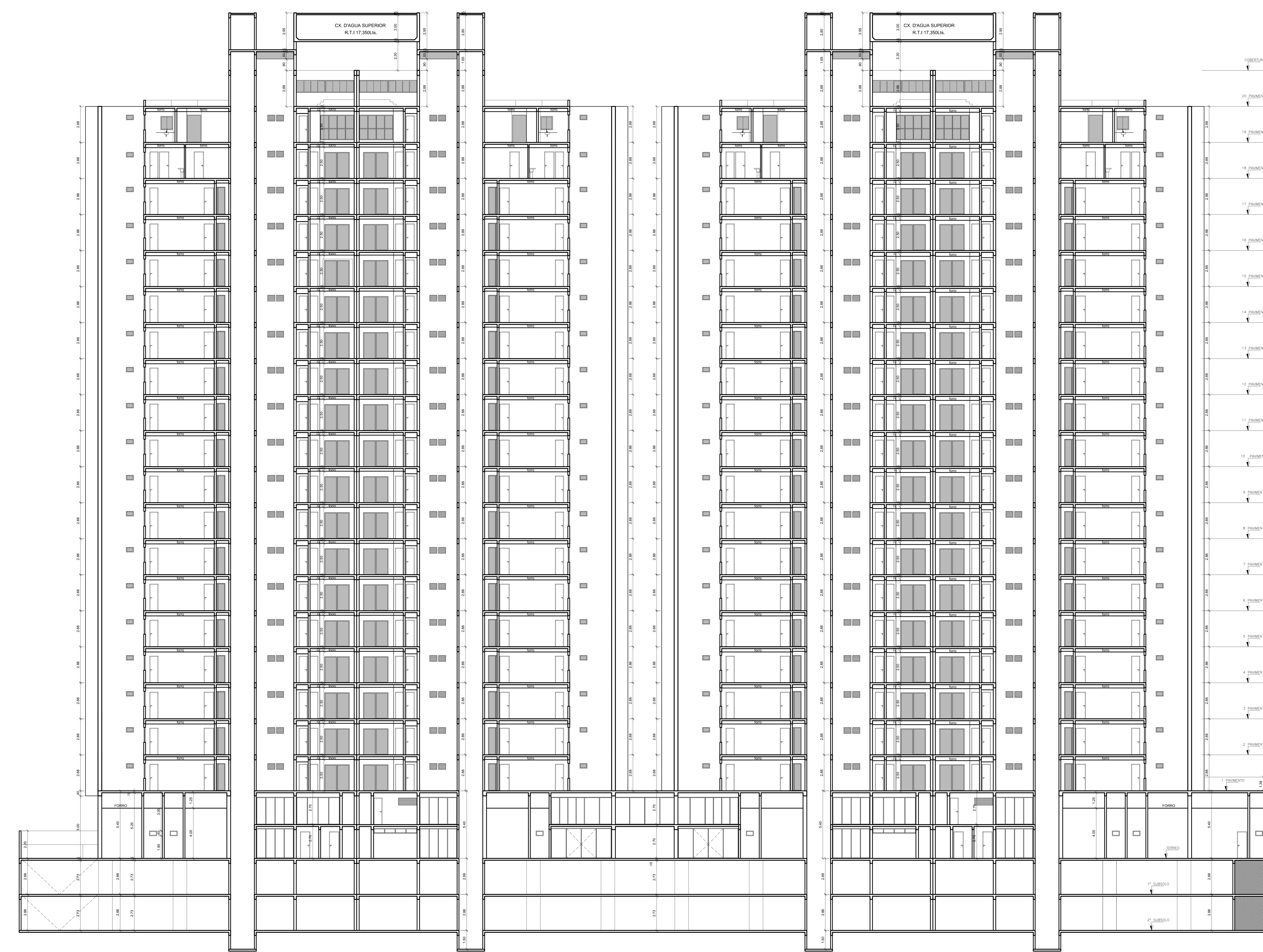
CORTE C-C ESCALA 1/10
